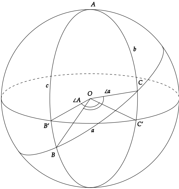
图 3.7: 球面上的角
