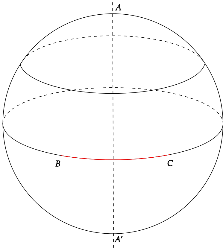
图 3.5: 大圆与小圆
